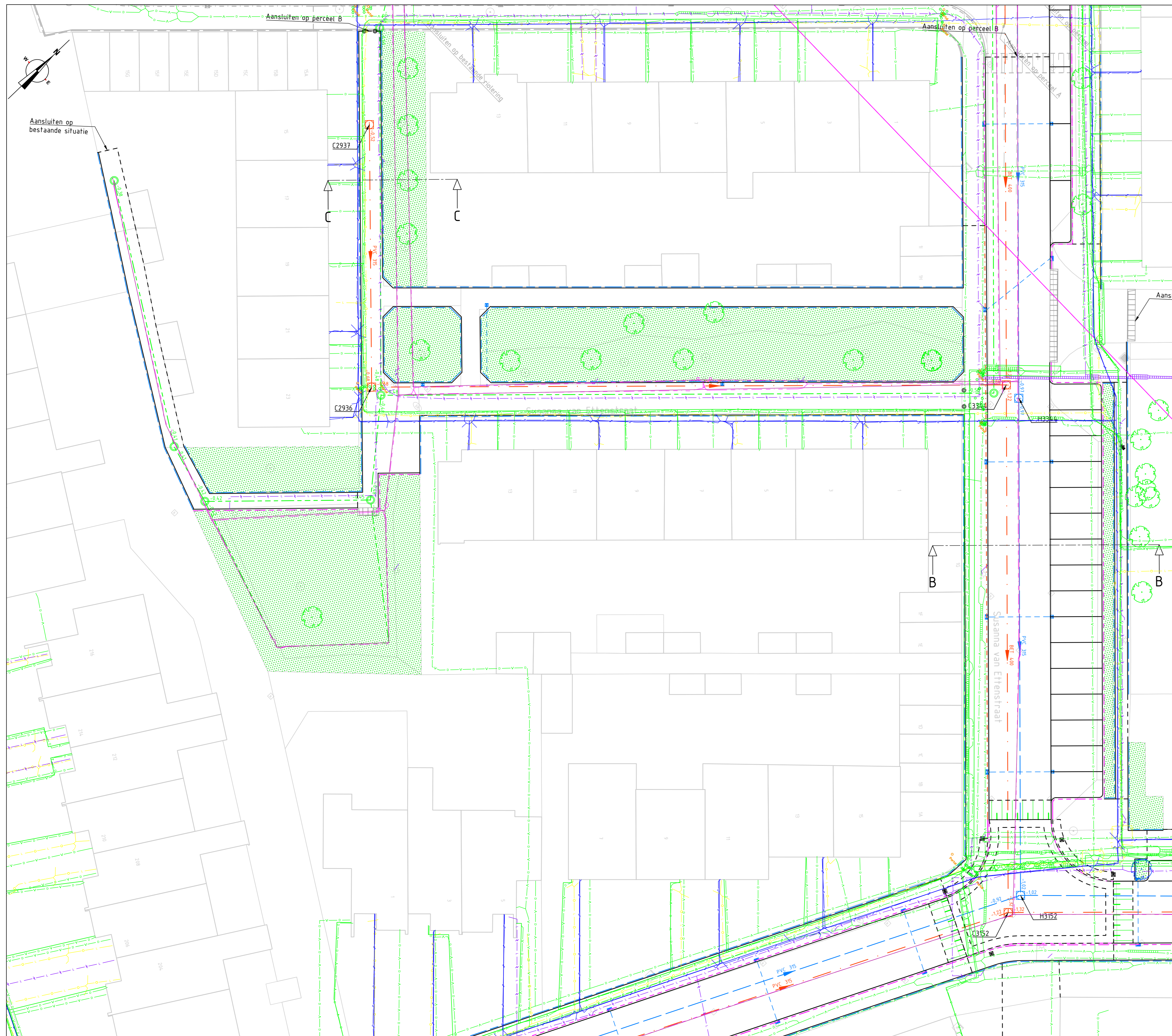
Bovenaanzicht 1B SCHAAL 1 : 200
