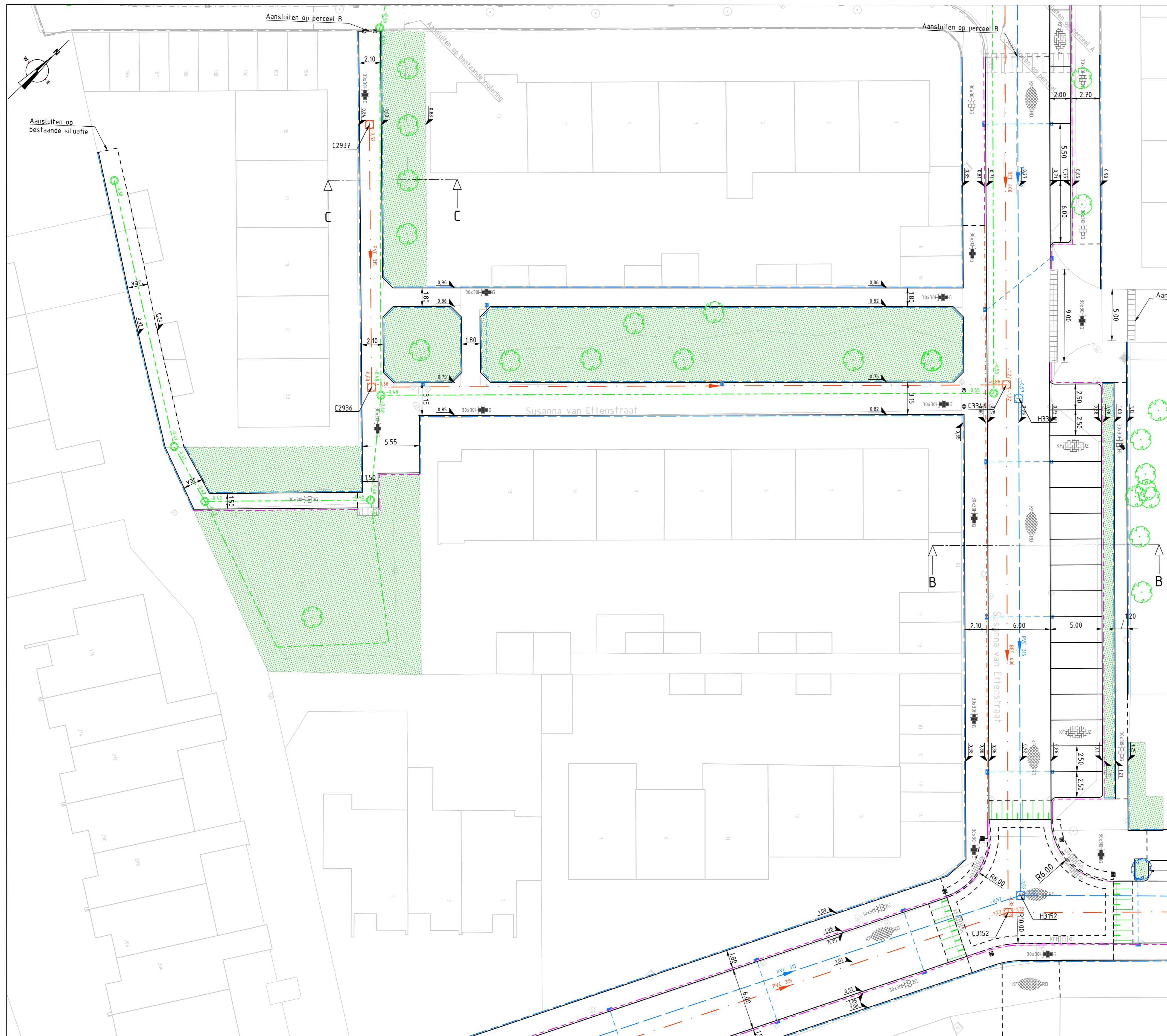
Bovenaanzicht 1B SCHAAL 1 : 200
