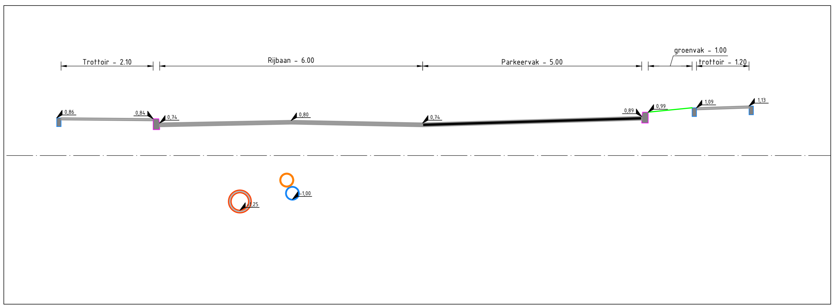
Doorsnede B-B Susanna van Effenstraat
