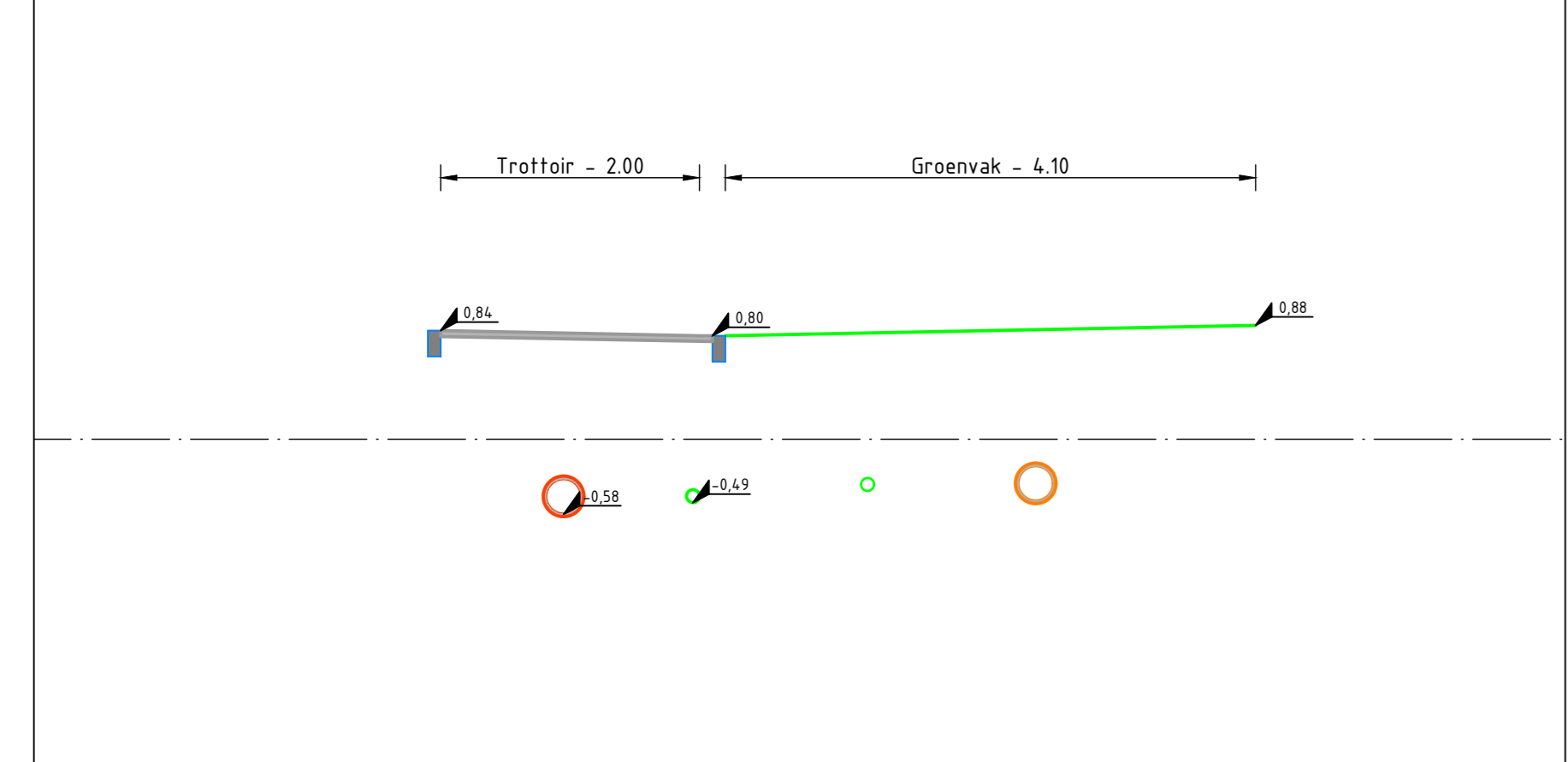
Doorsnede C-C Susanna van Effenstraat - hojje
