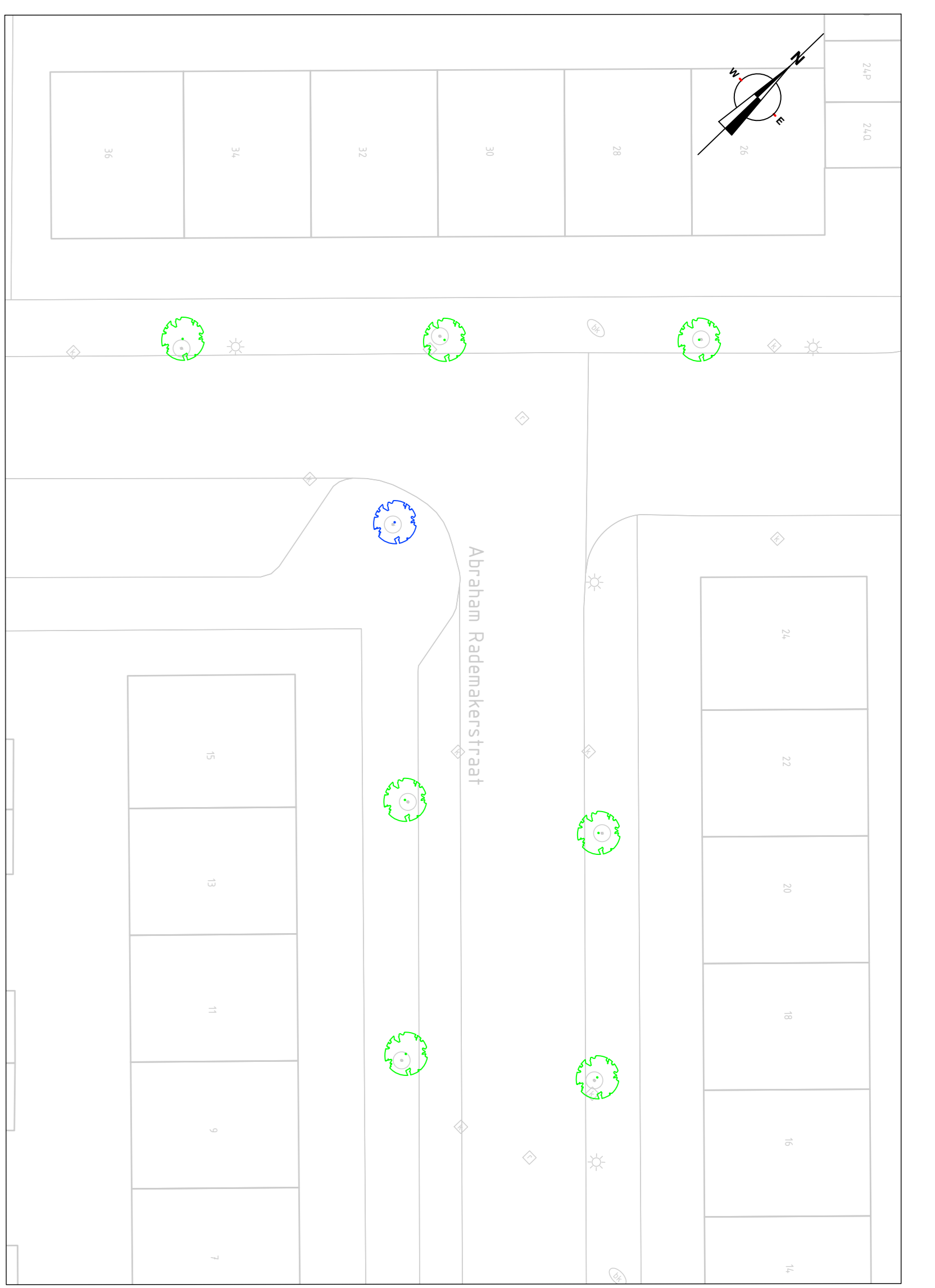
Bovenaanzicht 2 SCHAAL 1 : 200
