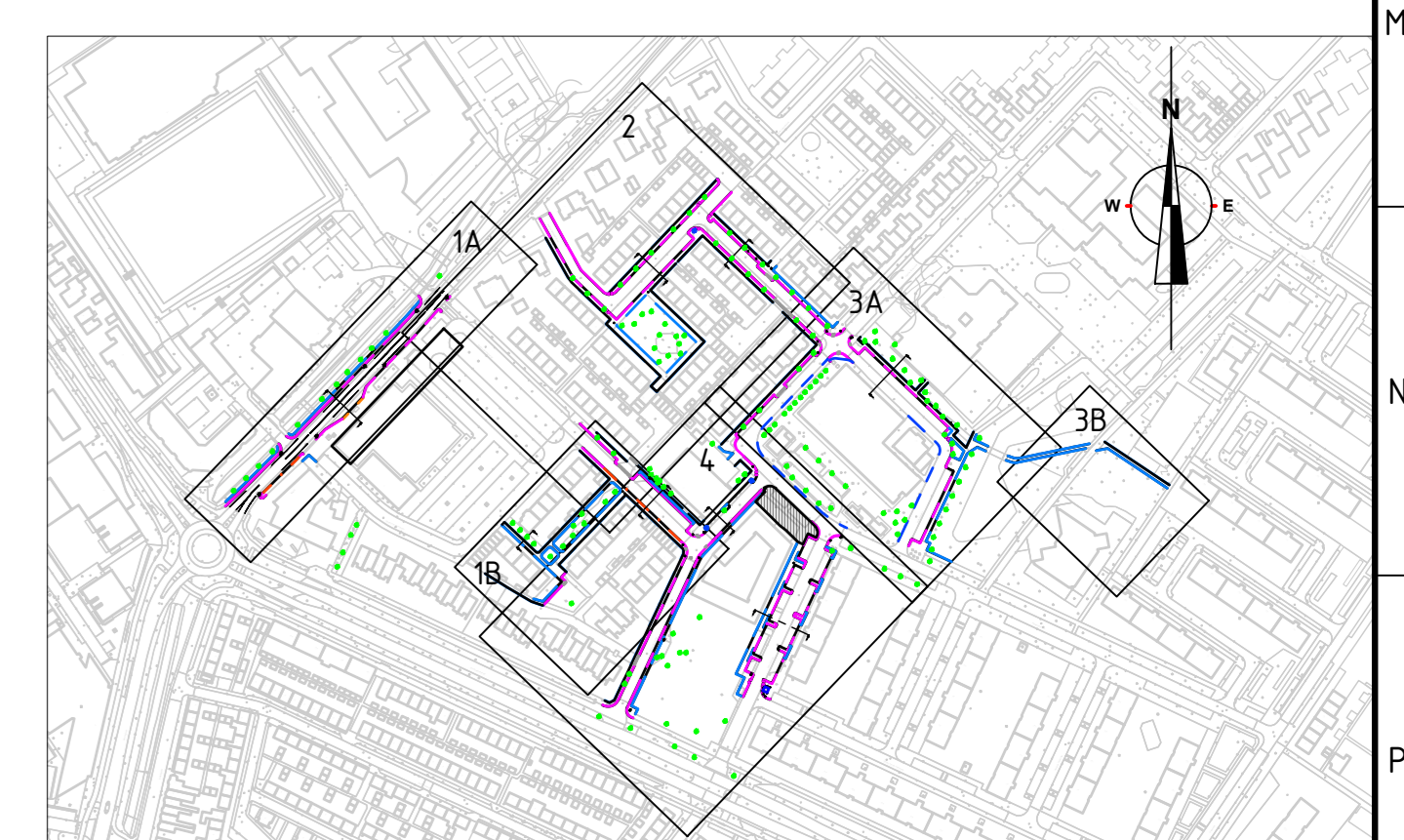
Overzicht SCHAAL 1:200
