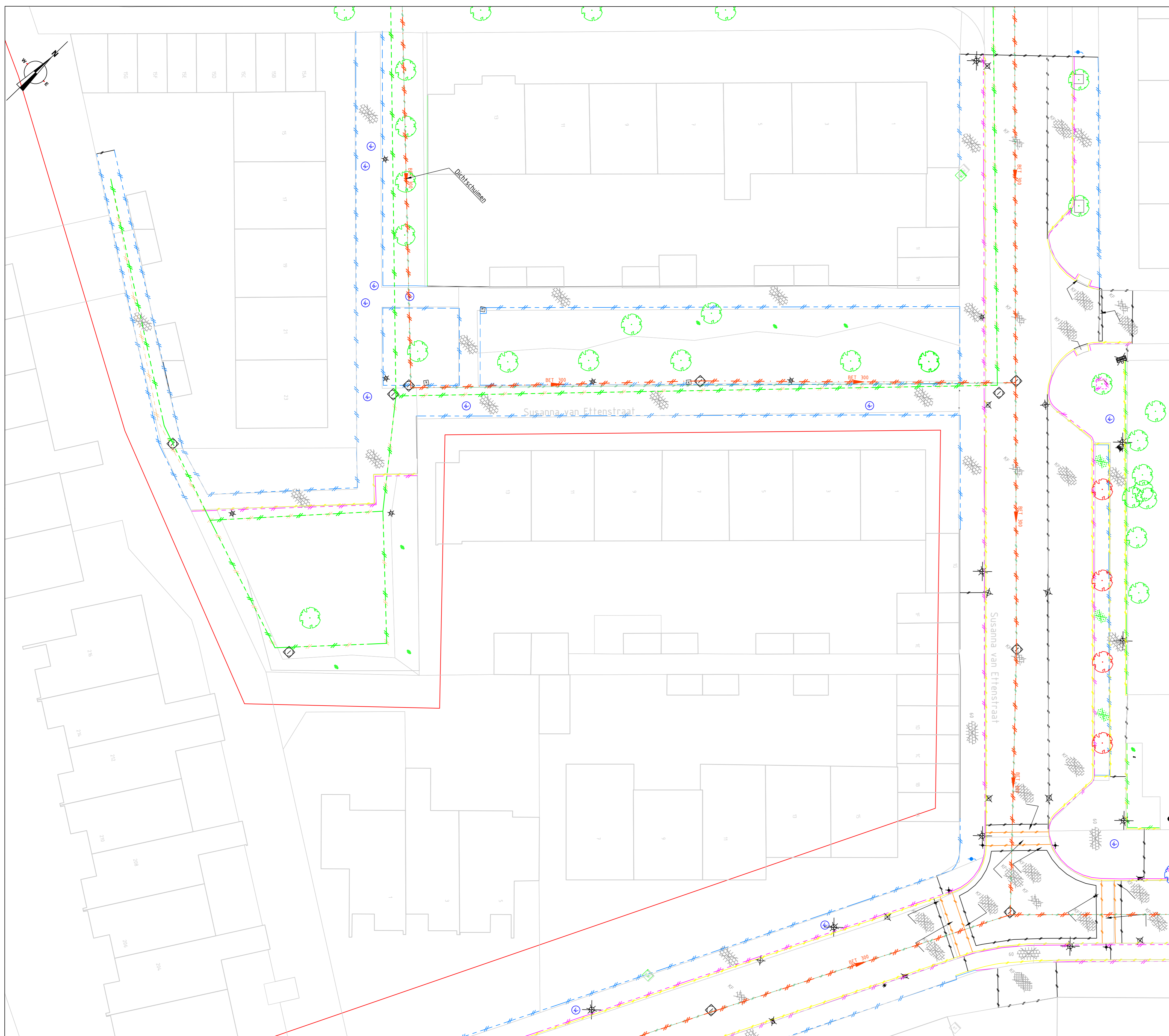
Bovenaanzicht 1B
