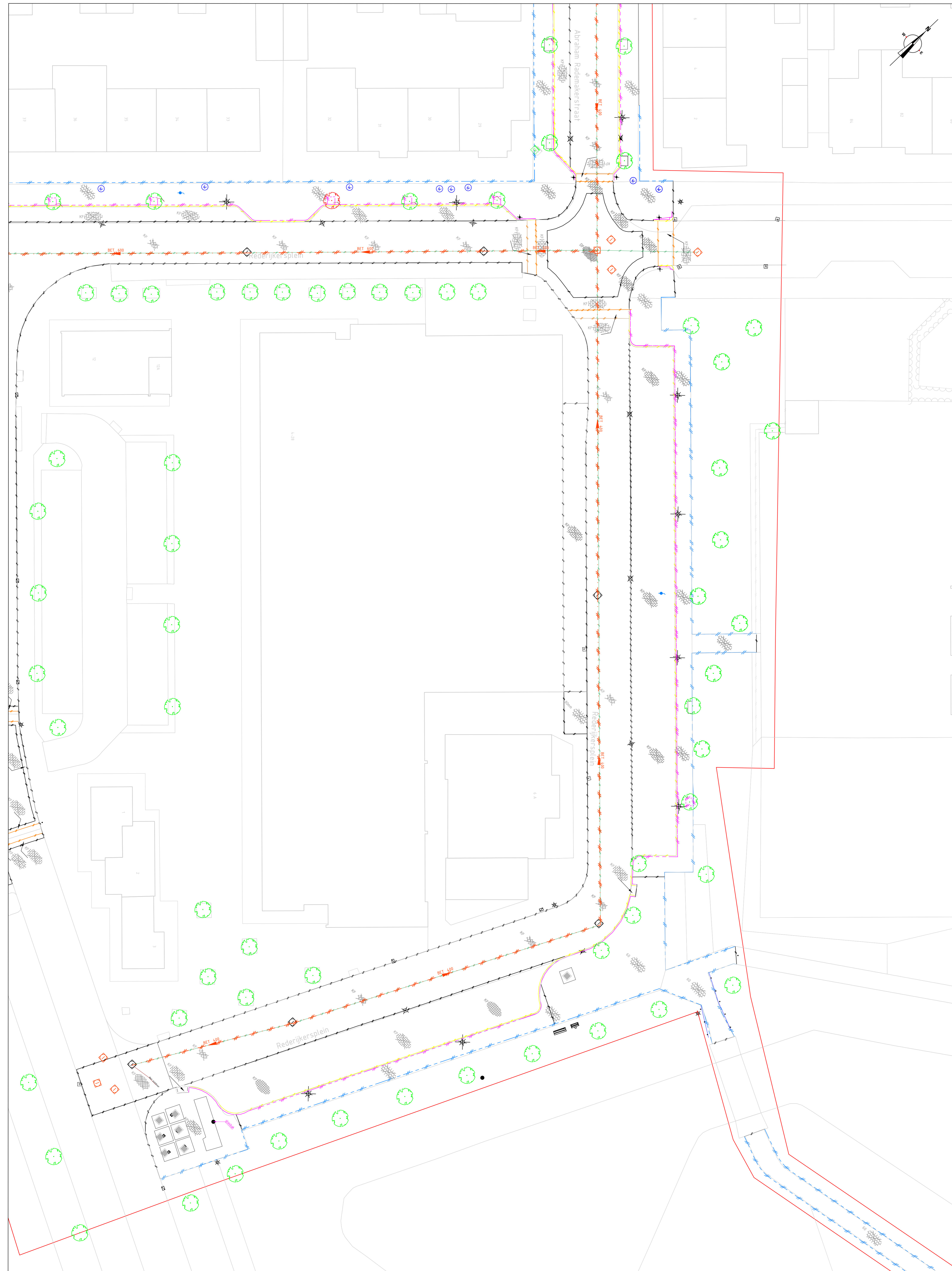
Bovenaanzicht 3A SCHAAL 1 : 200
