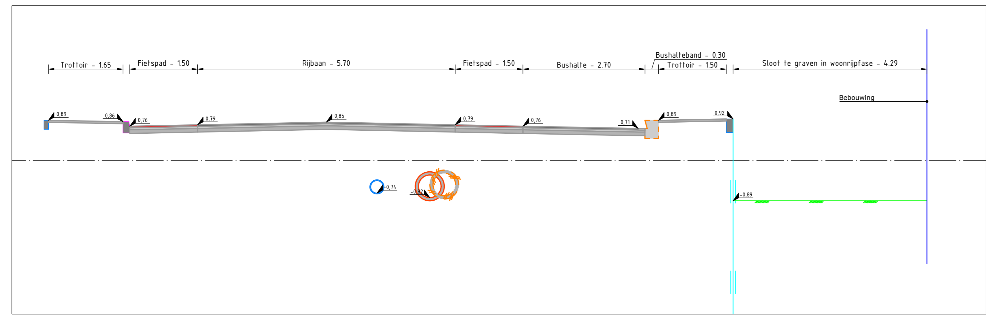
Doorsnede A-A Duinwetering
