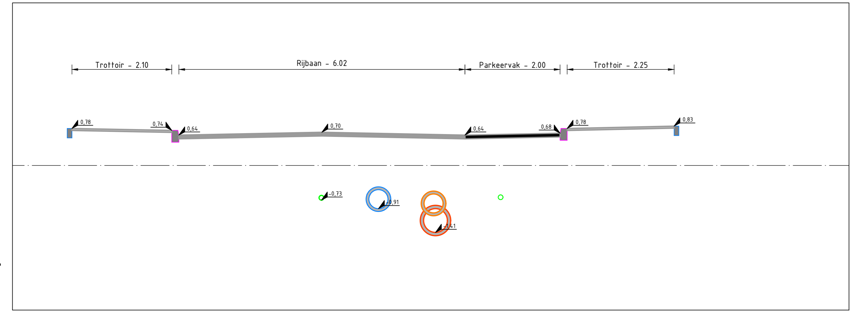
Doorsnede E-E Abraham Raaijmakerstraat 18
